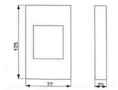
Instalar sobre caixa ou condutele 2x4, exceto modelo GC que pode ser instalado diretamente sobre a parede
